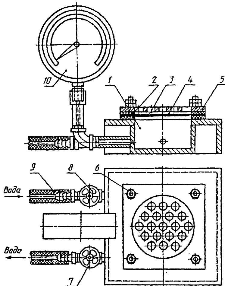
1 - рабочая камера; 2 - резиновые прокладки; 3 - образец; 4 - контактная сетка; 5 - прижимная плата; 6 - зажимные винты; 7, 8 - краны; 9 - резиновая трубка, соединяющая с водопроводом; 10 - манометр
