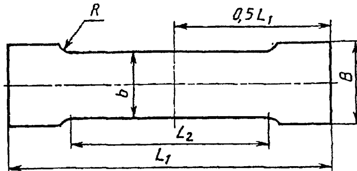
Рисунок 1. Образец-лопатка типа 1
