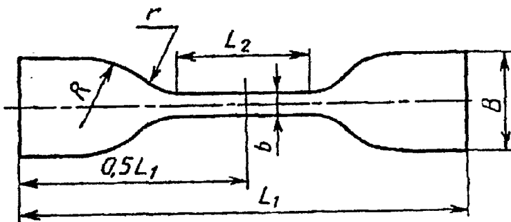
Рисунок 2. Образец-лопатка типа 2
